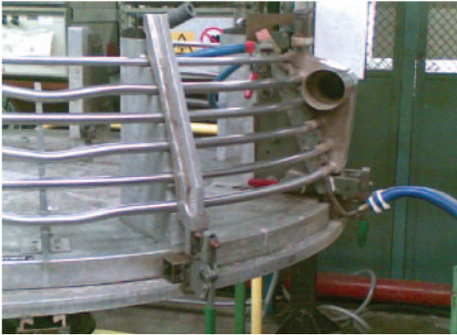
Brasage de conduite de fluide
